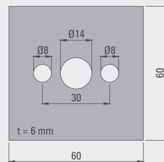
Verfüllscheibe M12 für Befestigungsmittel Ø12 mm
