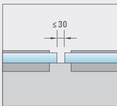
2 Glasstoß
