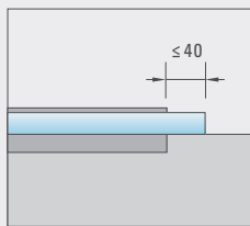
3 Glasüberstand
