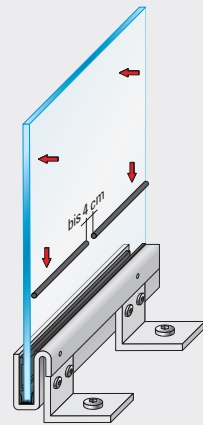
6 POM-Stab (rund) einsetzen. Glas nach außen drücken, POM-Stab eindrücken und mit Setzwerkzeug einschlagen.
