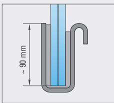
1 Glaseinstand
