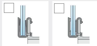
Keilsystem
