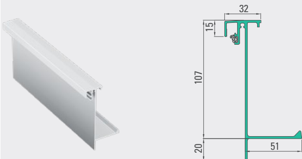
Unteres Profil BVU-A
